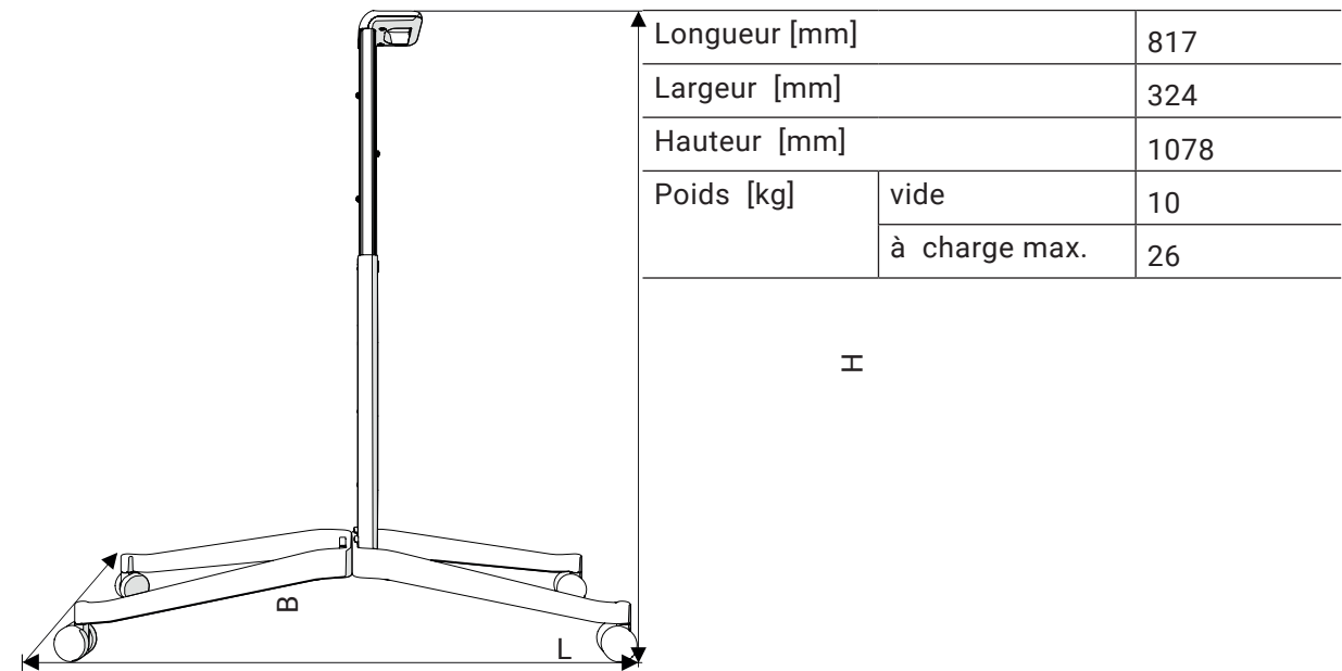
Fig. 2 Dimensions du Caddy de bureau Meeting
